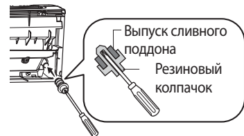
Сливной шланг
