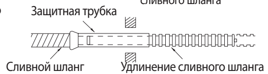
Отверстие для сливного шланга
