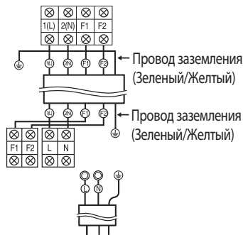
Внутренний блок
