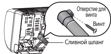
Выпуск сливного поддона
