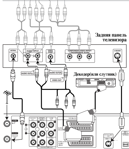
Задняя стенка прибора (простое соединение)
