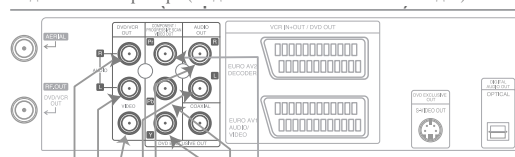
Задняя стенка прибора (Подключение компонентного видео)
