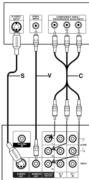
Задняя панель DVD/CD ресивера
