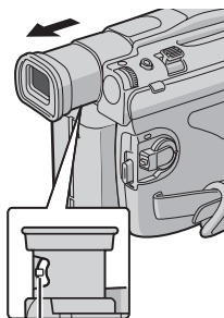
Регулятор диоптра
