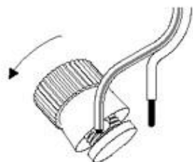
Рис. 4. Закрыть зажим
