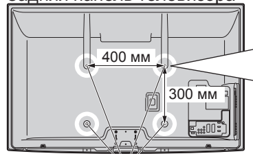
Отверстия для крепления настенного кронштейна
