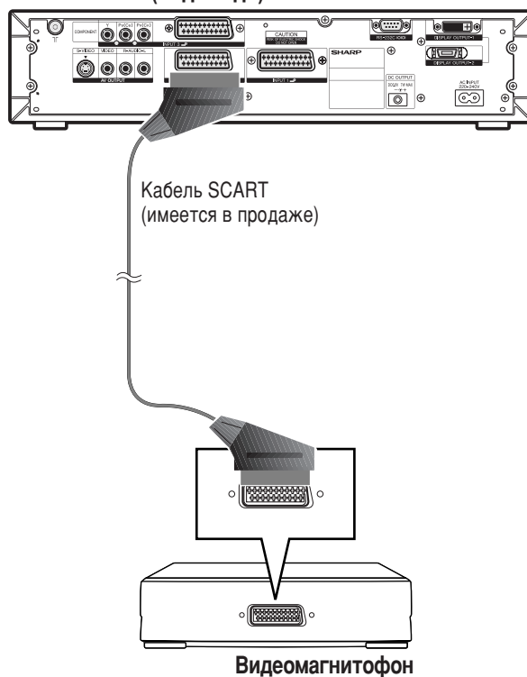
Система AVC (вид сзади)
