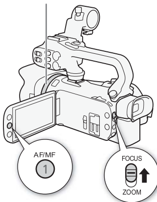
Кольцо фокусировки/зумирования
