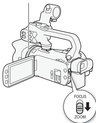
Кольцо фокусировки/зумирования
