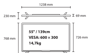
Габаритные размеры, размер настенного крепления, вес | Overall dimensions, wall attachment size, weight
