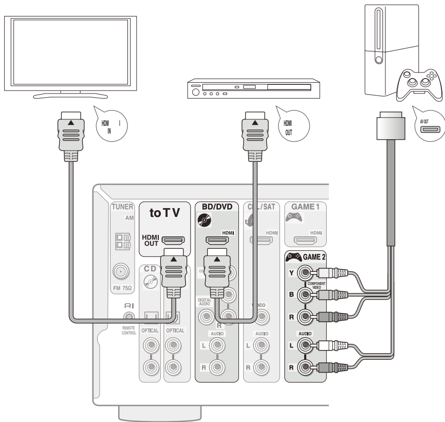
Пример соединений
