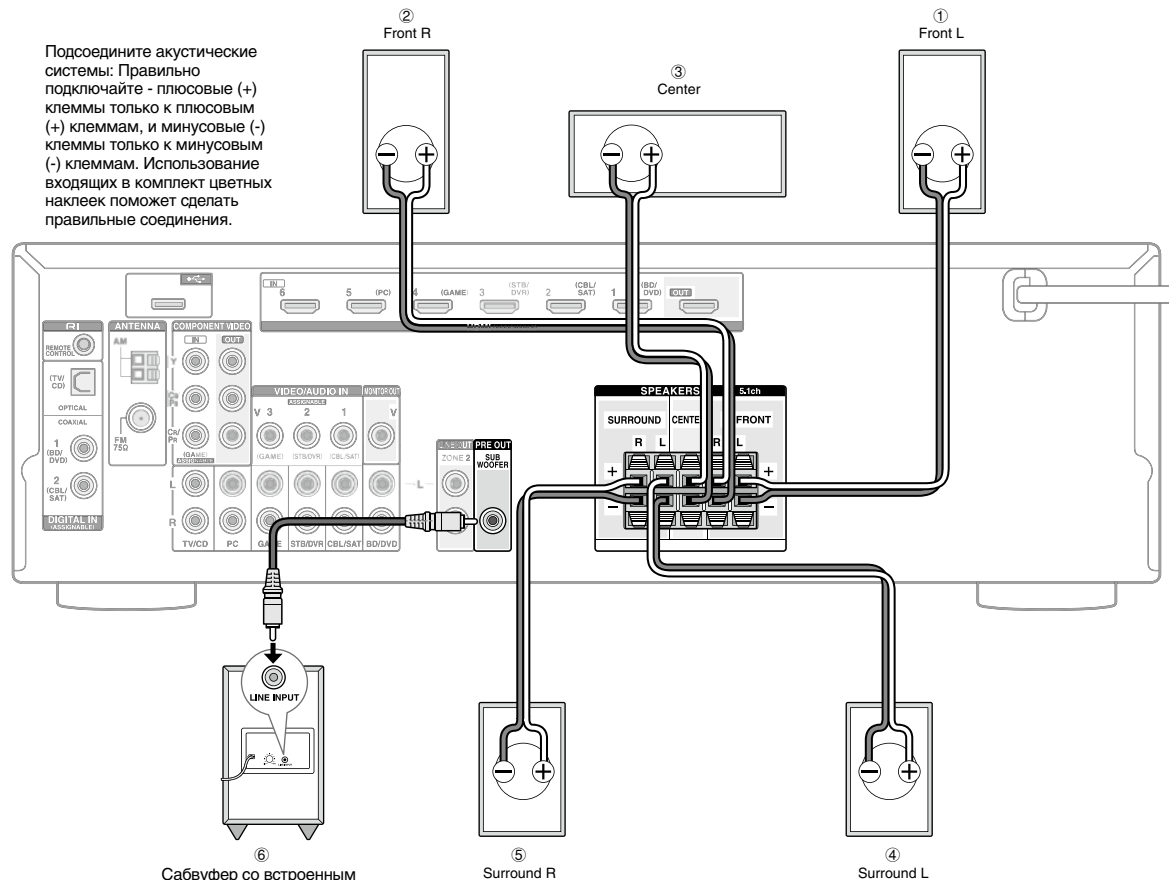
⑥ Сабвуфер со встроенным усилителем мощности.
