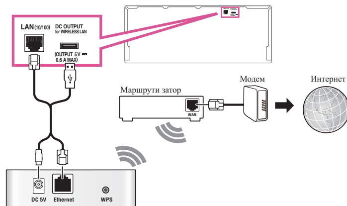
Адаптор беспроводной сети LAN (AS-WL300)
