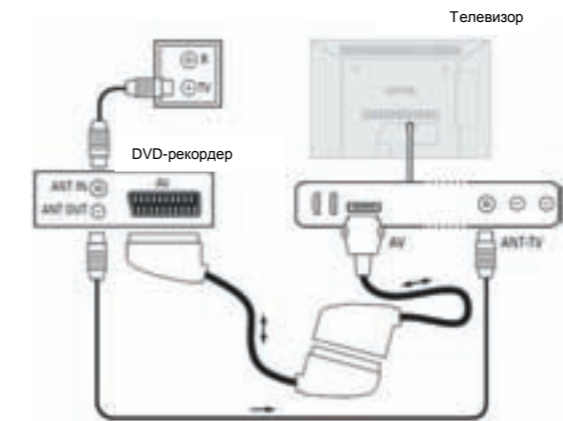
Пример подключения DVD-рекордера
