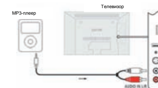
Аудиовход – левый/правый канал Пример подключения MP3-плеера
