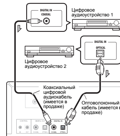
Задняя панель PD-50
