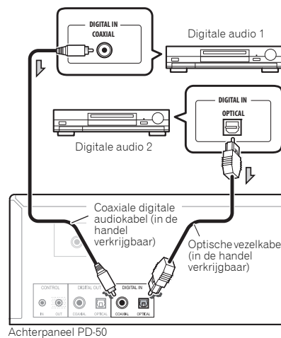
Achterpaneel PD-50
