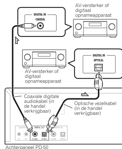
Achterpaneel PD-50
