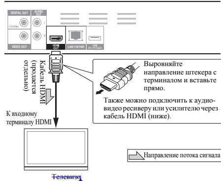
Задняя панель проигрывателя
