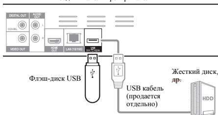
Задняя панель проигрывателя
