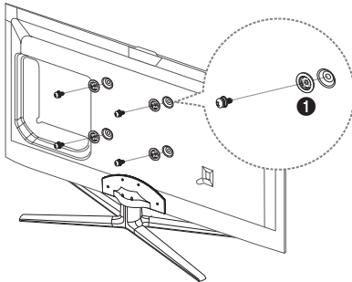
Вариант А. Установка настенного крепления SAMSUNG
