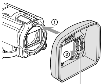
Фиксирующее кольцо
