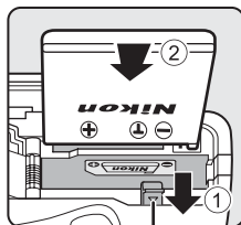
Защелка батареи
