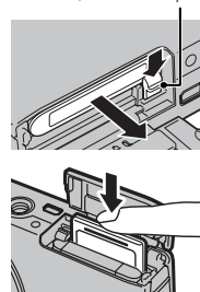
Защелка батареи
