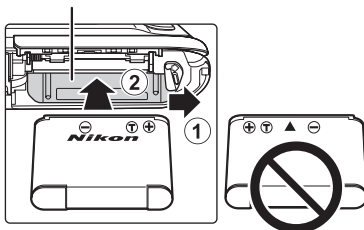
Батарейный отсек
