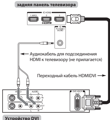
Устройство DVI
