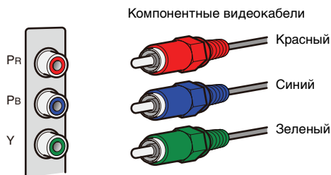
Компонентные видеокабели
