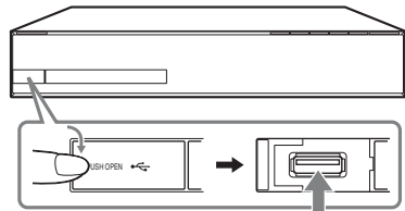
Пристрій USB
