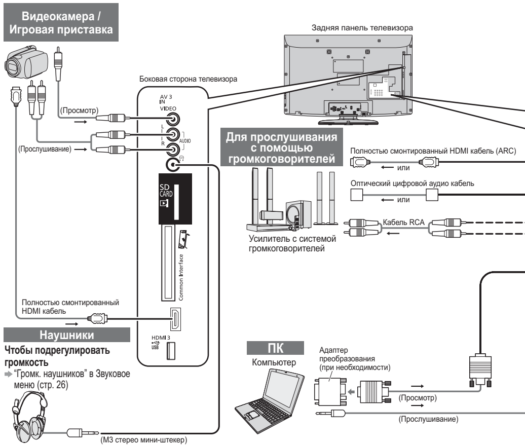
Типы оборудования, которое можно подсоединить к каждому разъему
